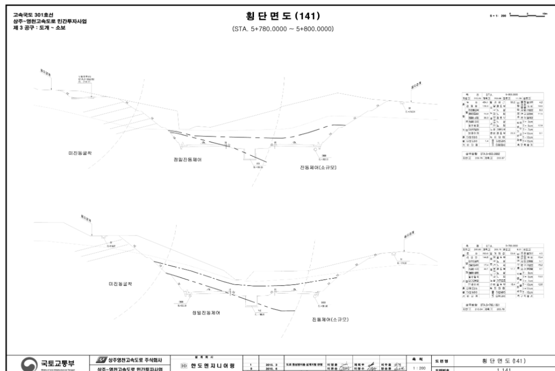
【그림 17.1.5】 표준횡단면도
